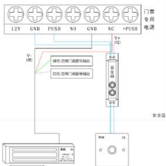
井田JT-6000防爆电磁锁单锁系统配置图
